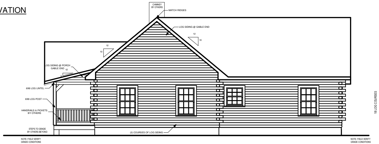
RIGHT ELEVATION
