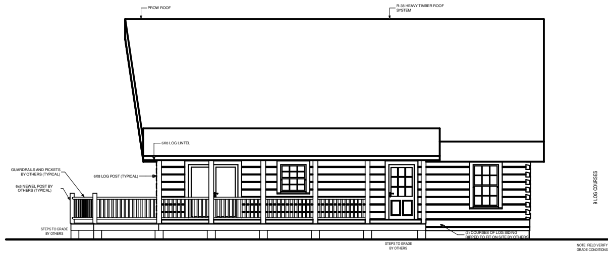
RIGHT ELEVATION
